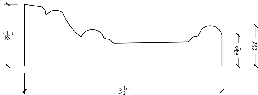
CASING SCALE: 1'-0"=1'-0"
