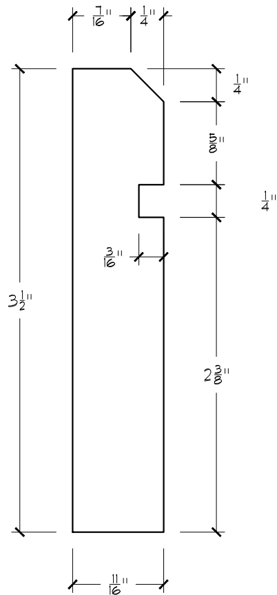
CASING SCALE: 1'-0"=1'-0"
